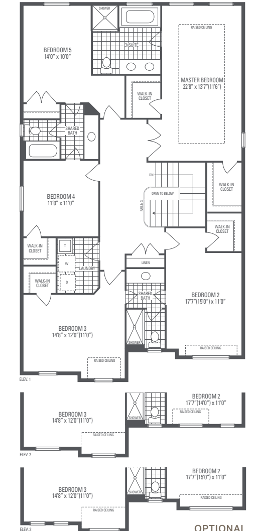
OPTIONAL 5 BEDROOM UPPER LEVEL
