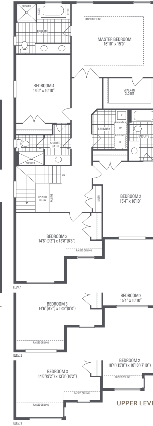
OPTIONAL 3 ENSUITE UPPER LEVEL
